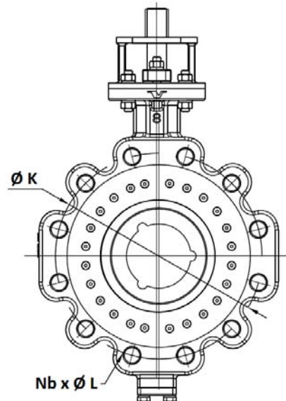
DN200
