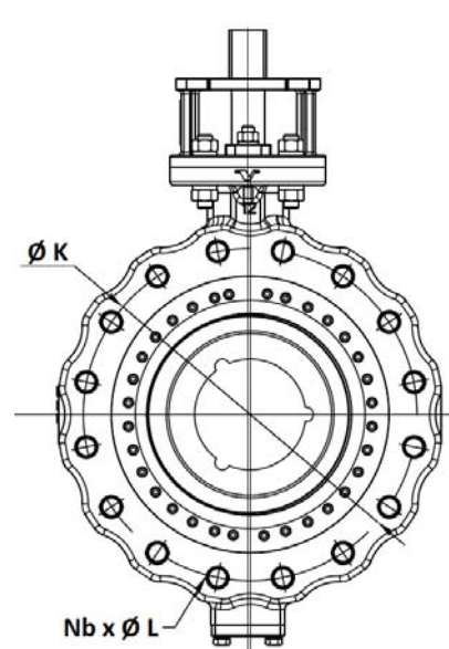
DN300
